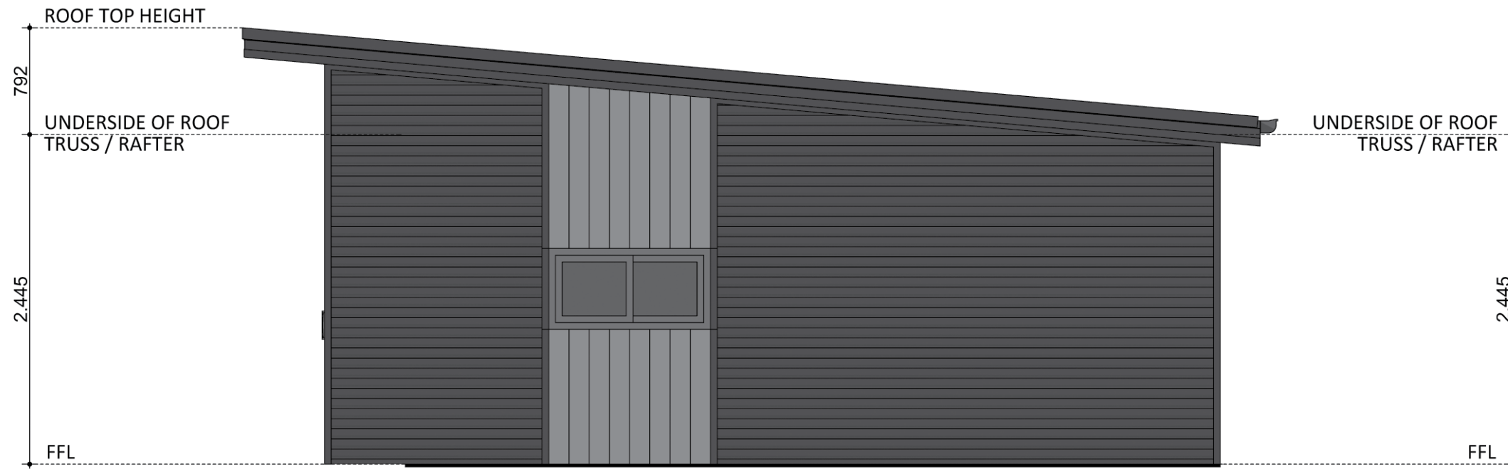
ELEVATION 02
