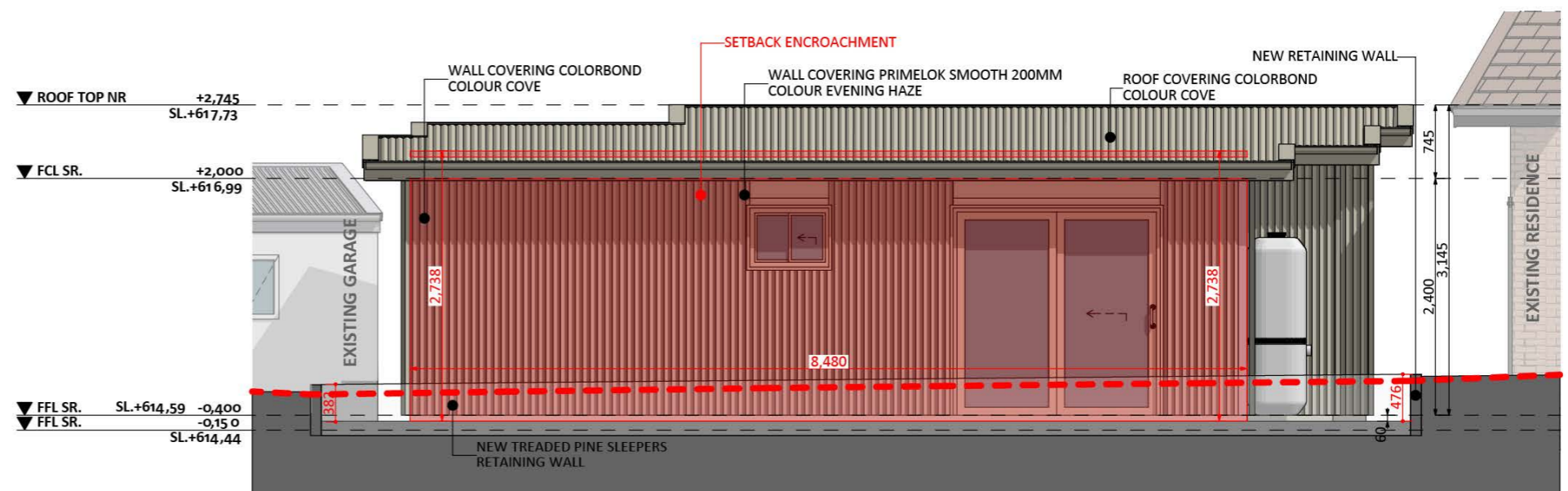
ELEVATION 02
