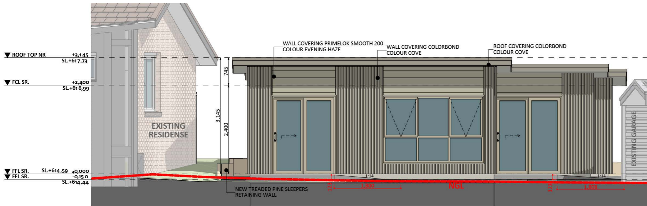
ELEVATION 01
