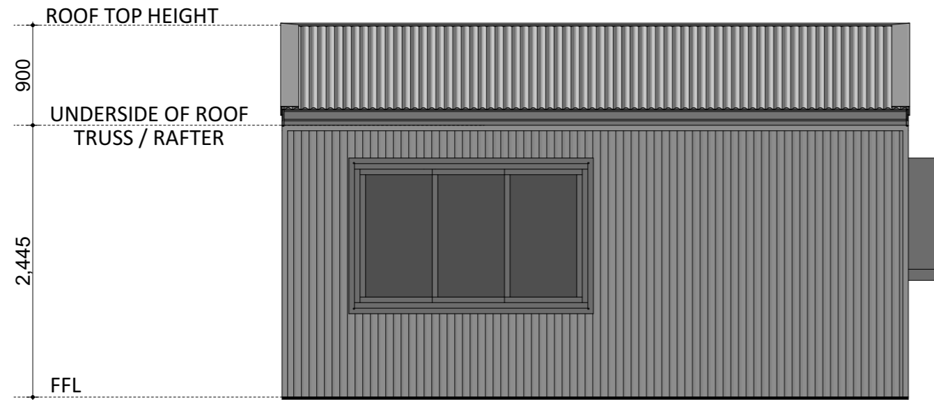
ELEVATION 3
