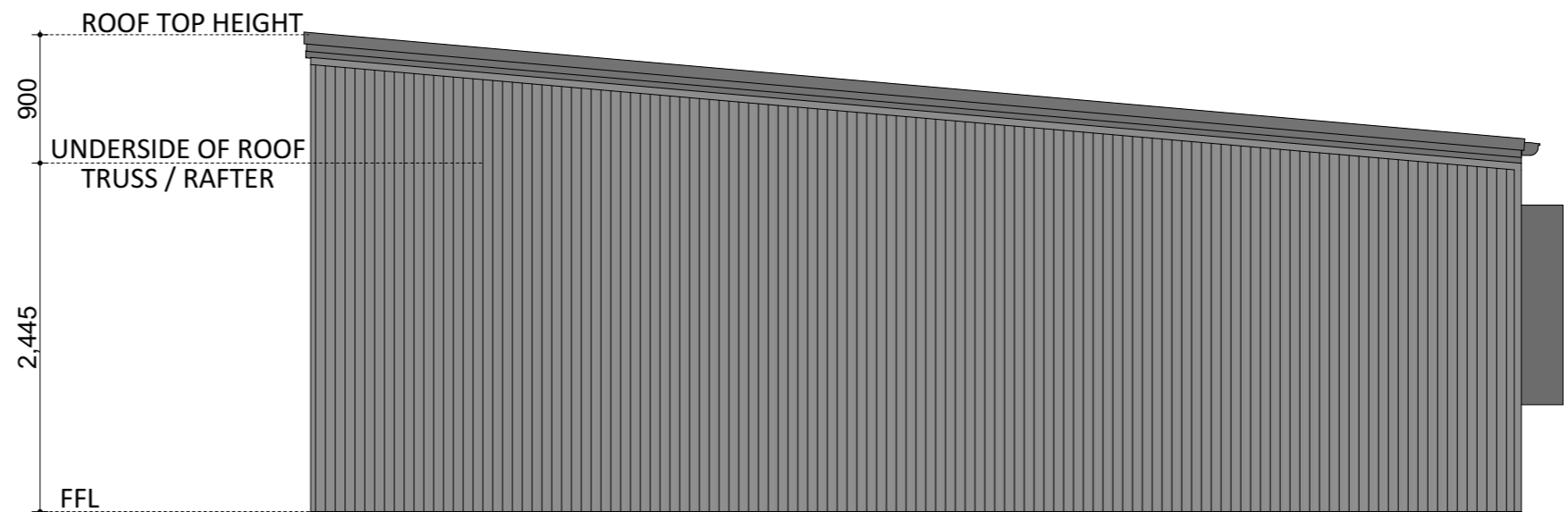
ELEVATION 4
