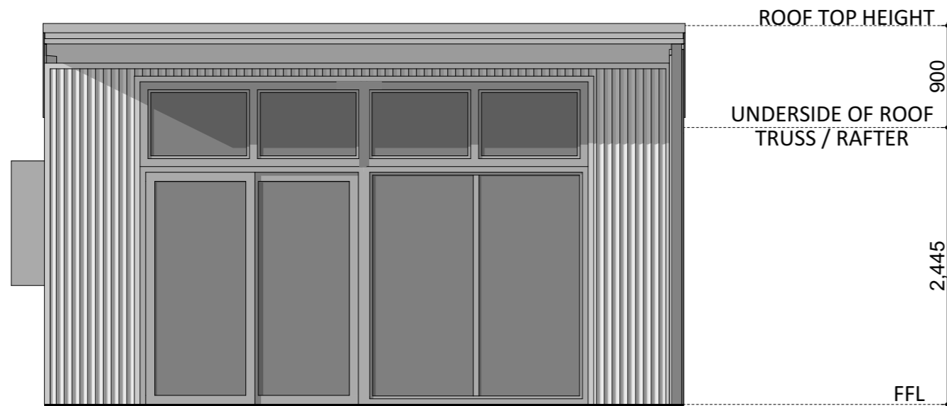
ELEVATION 1
