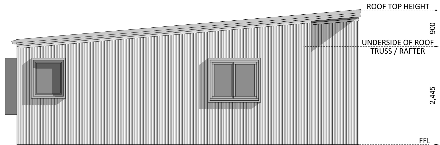
ELEVATION 2
