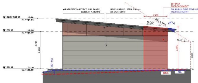
ELEVATION 02
